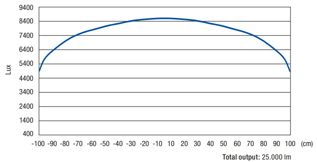
P12 Lichtverteilung
