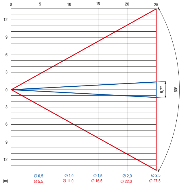
P12 Abstrahlwinkel
