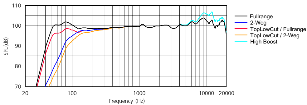
Frequenzgang ‚on axis‘ mit K&F Controller C2 (Filters ‚OFF‘)
