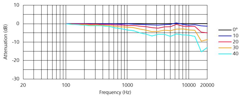
Horizontaler Frequenzgang ‚off axis‘
