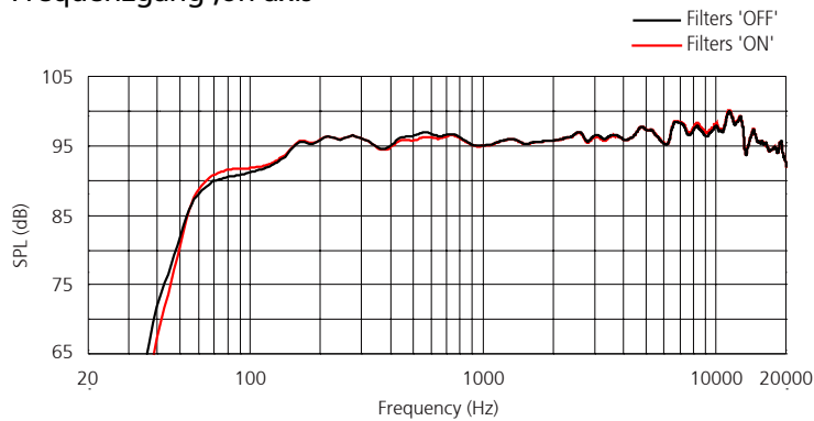
Frequenzgang ‚on axis‘
