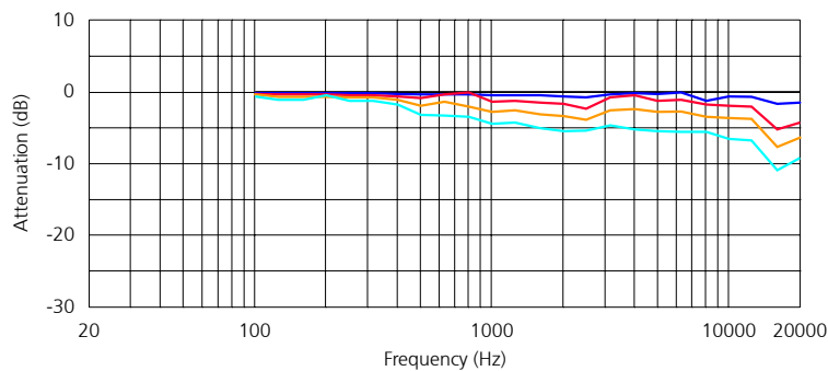
Horizontaler Frequenzgang ‚off axis‘
