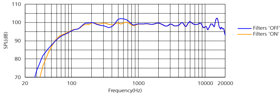
Frequenzgang ‚on axis‘
