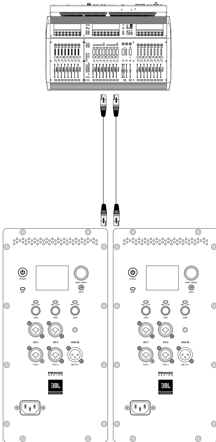
ZWEI SYSTEME WERDEN ALS MONITORE VERWENDET PRX900 links und PRX900 rechts
