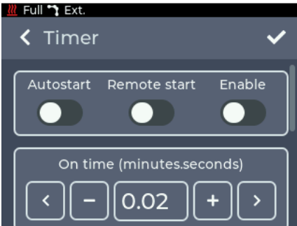
Abb. 19: Einstellungen Timer
