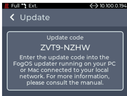
Abb. 36: Menü Update
