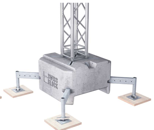
Ausleger ausgezogen
